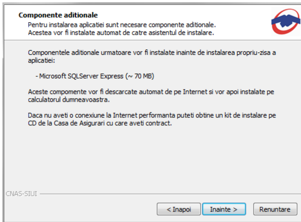
Figura 4.7 Confirmarea instalării - 1
