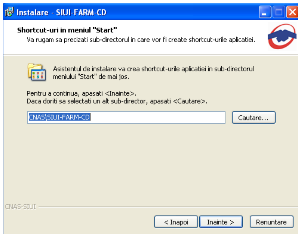
Figura 4.6 Alegerea shortcut-ului
