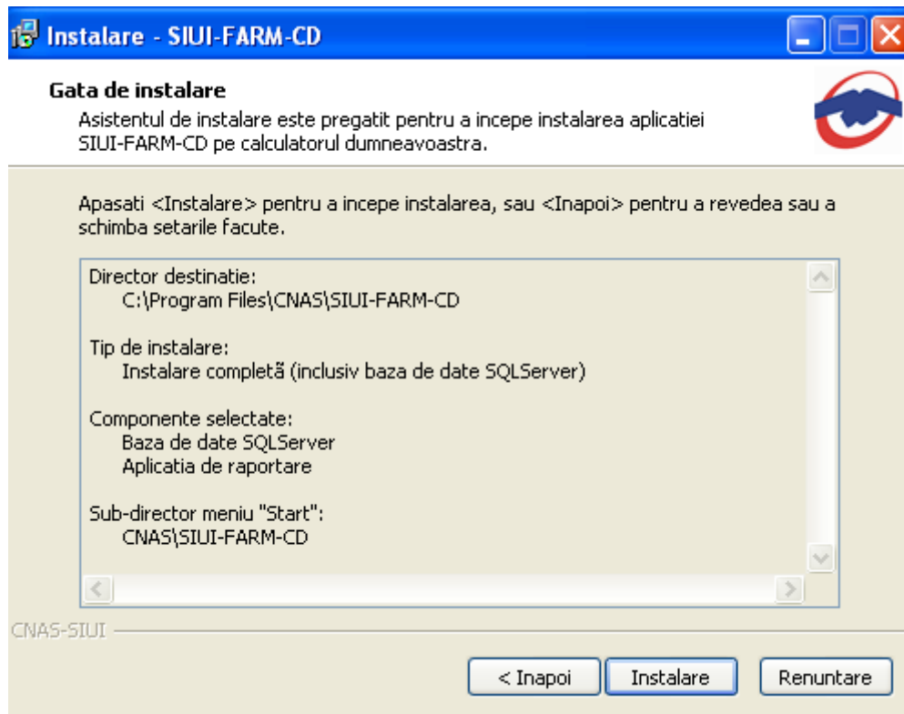
Figura 4.8 Confirmarea instalării - 2
